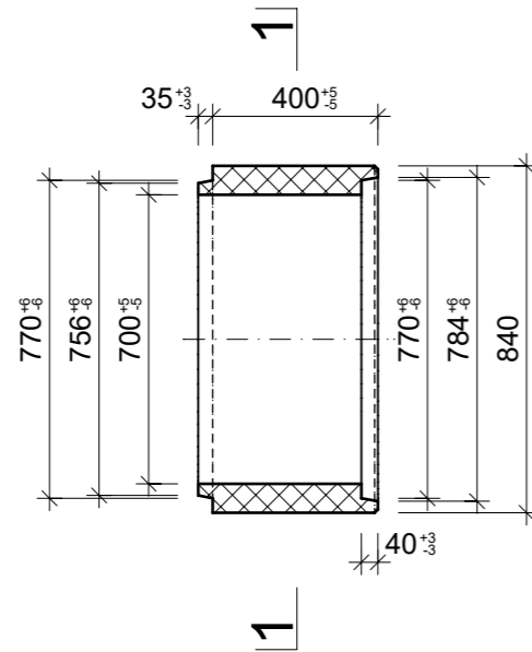
Grundriss, 1:20
