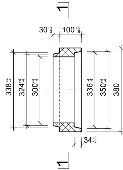
Grundriss, 1:10
