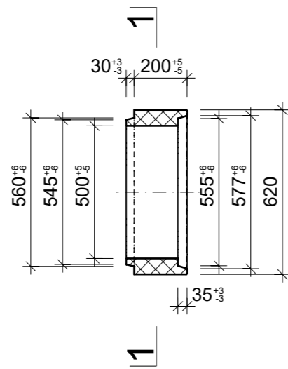
Grundriss, 1:20
