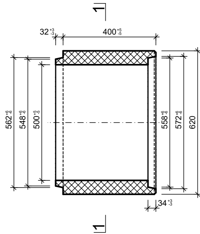
Grundriss, 1:10
