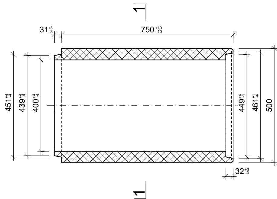
Grundriss, 1:10
