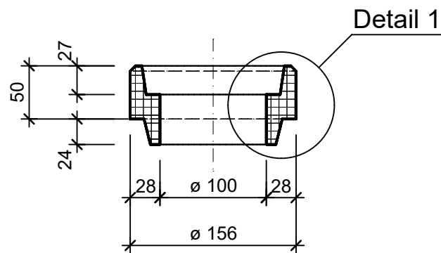
Schnitt A - A, 1:5
