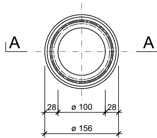
Grundriss, 1:5
