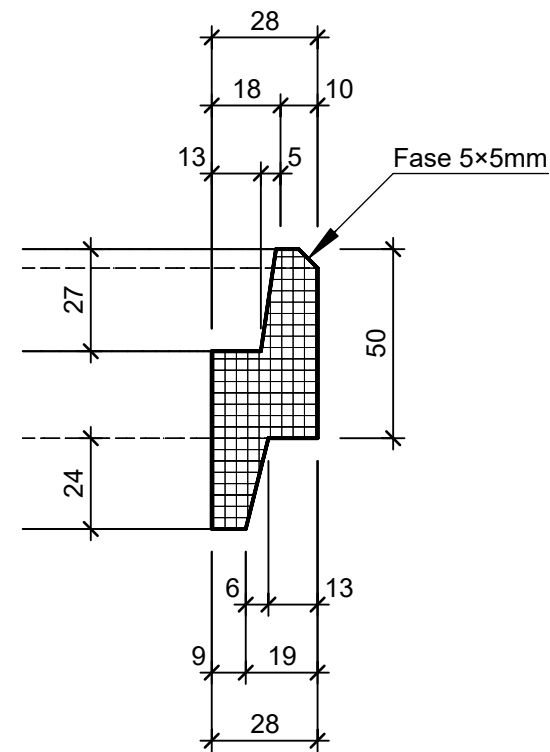
Detail 1, 1:2
