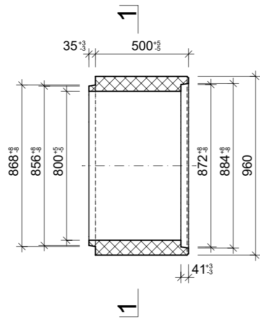
Grundriss, 1:20
