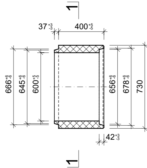
Grundriss, 1:20
