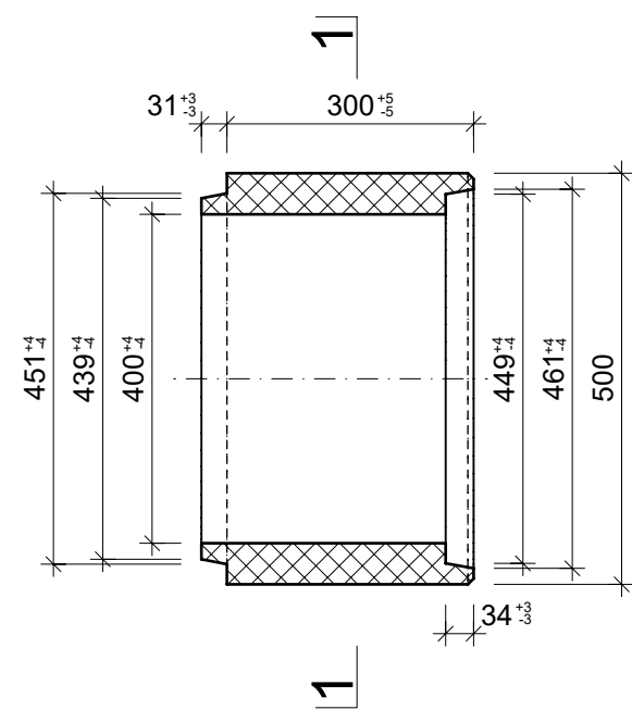
Grundriss, 1:10
