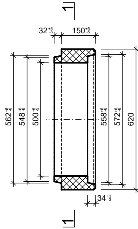
Grundriss, 1:10
