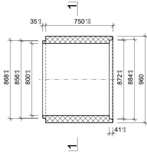
Grundriss, 1:20
