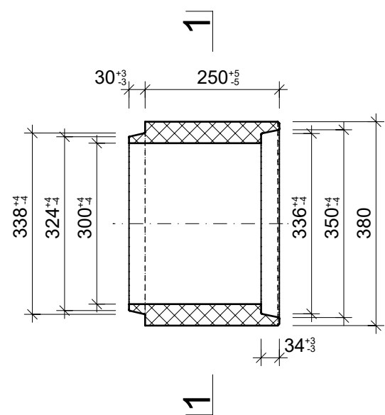
Grundriss, 1:10
