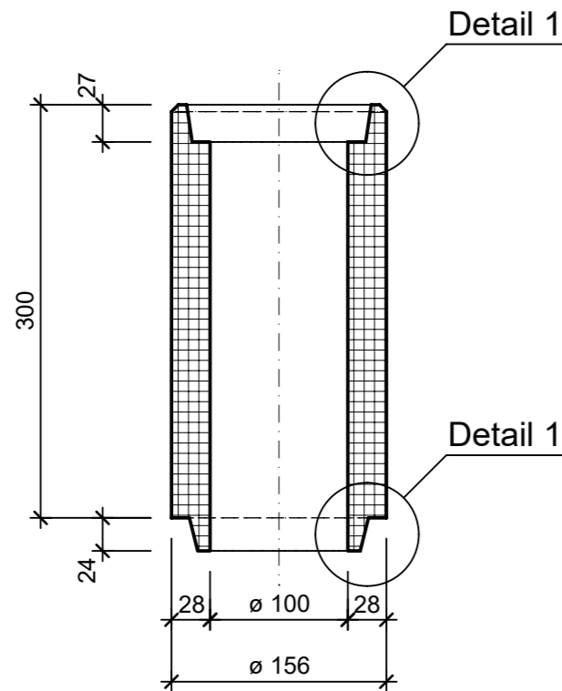
Schnitt A - A, 1:5
