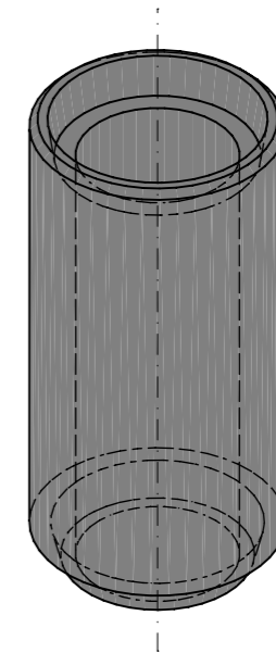
Isometrie, 1:5
