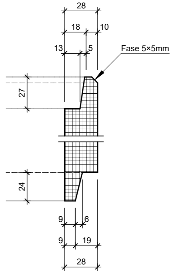
Detail 1, 1:2
