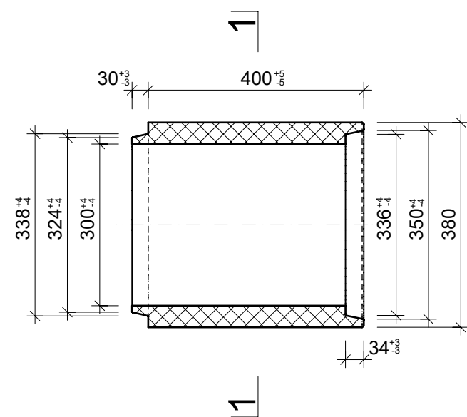
Grundriss, 1:10
