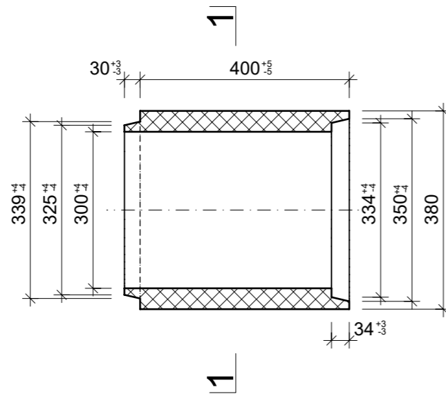
Grundriss, 1:10
