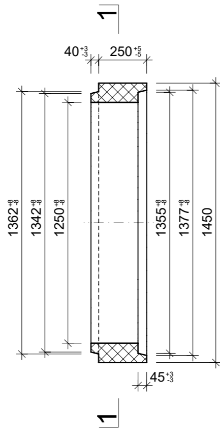
Grundriss, 1:20
