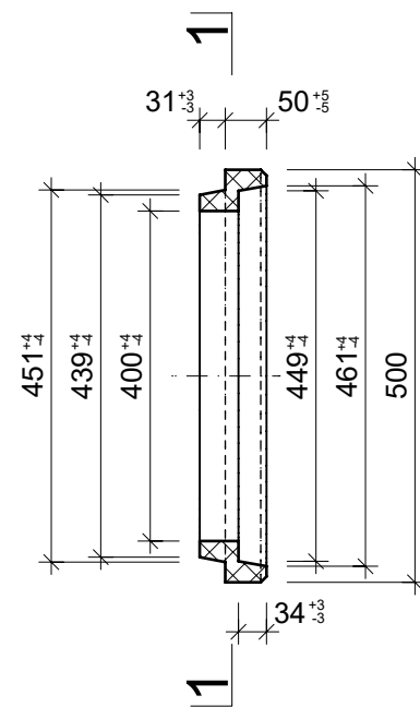
Grundriss, 1:10
