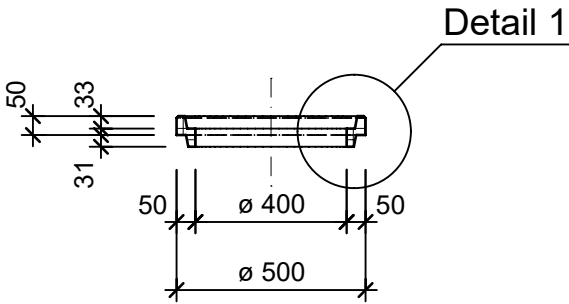
Schnitt A - A, 1:20
