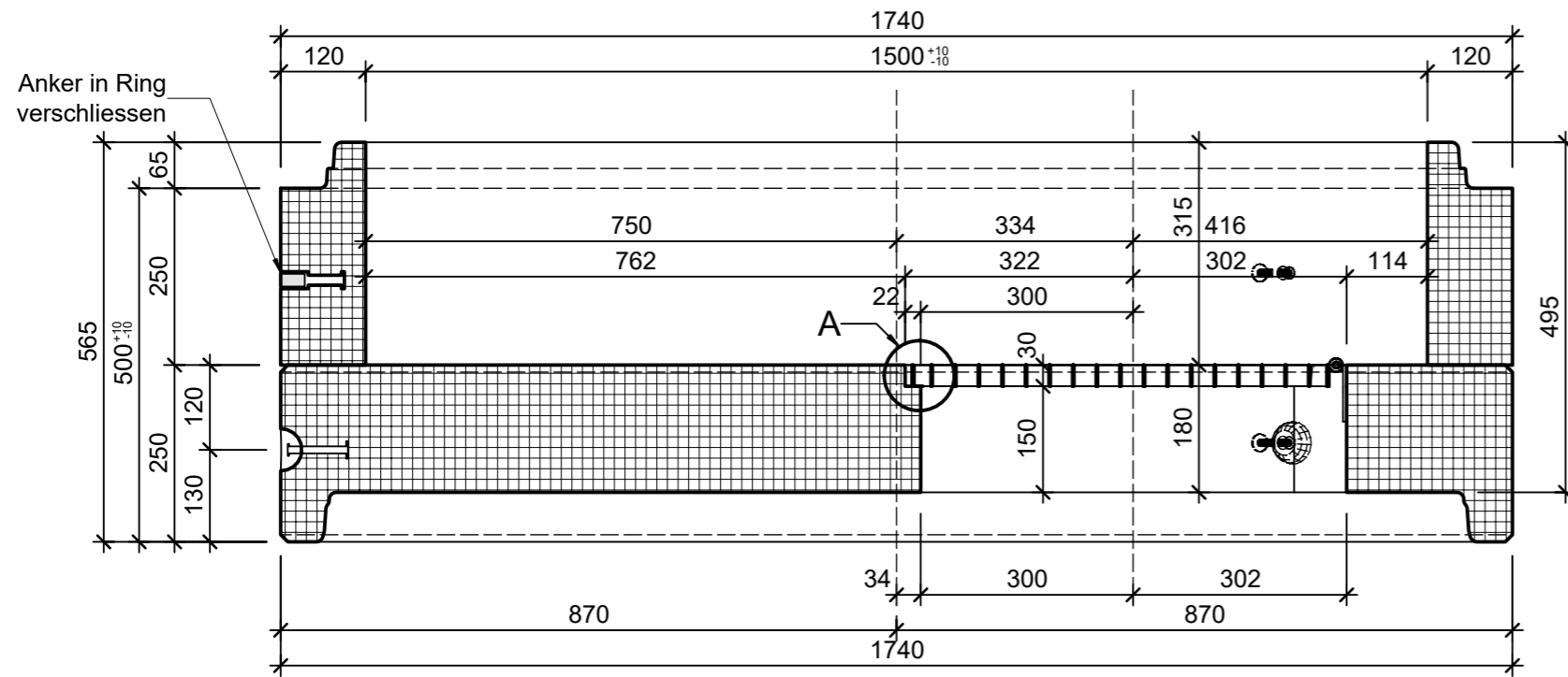
Grundriss 1:20
