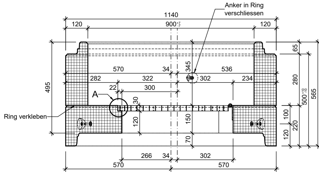
Schnitt 1, 1:10
