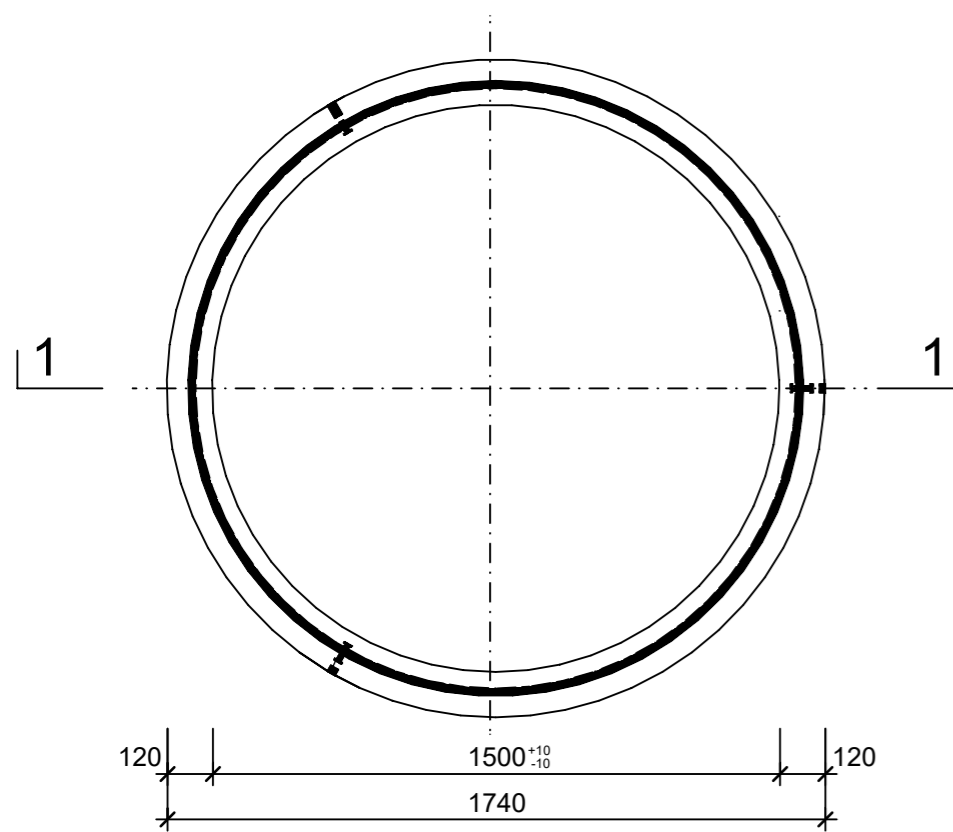
Grundriss, 1:20
