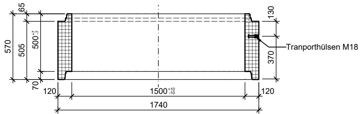
Schnitt 1-1, 1:20
