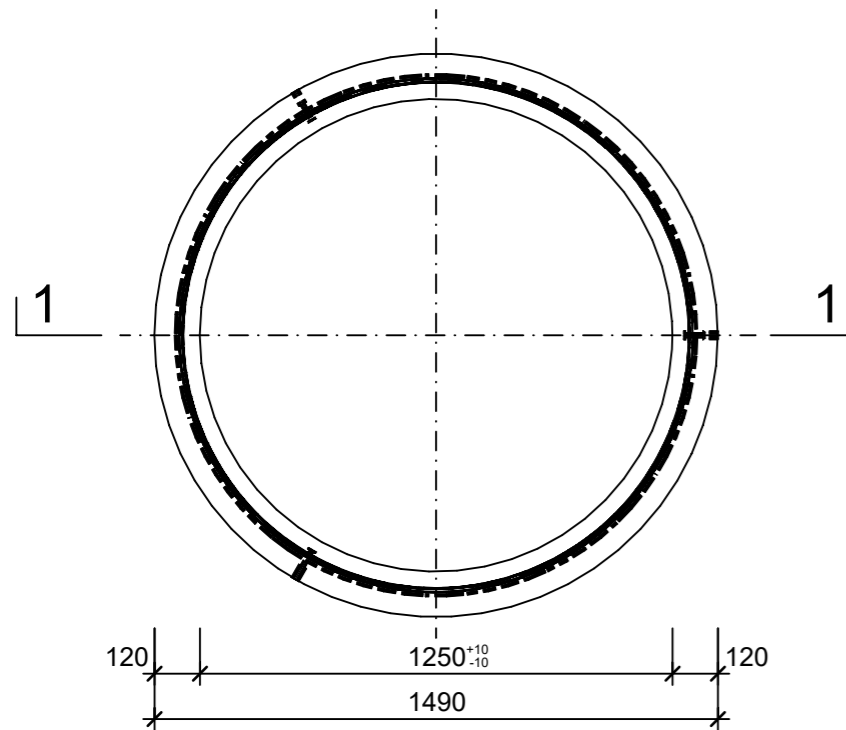
Grundriss, 1:20
