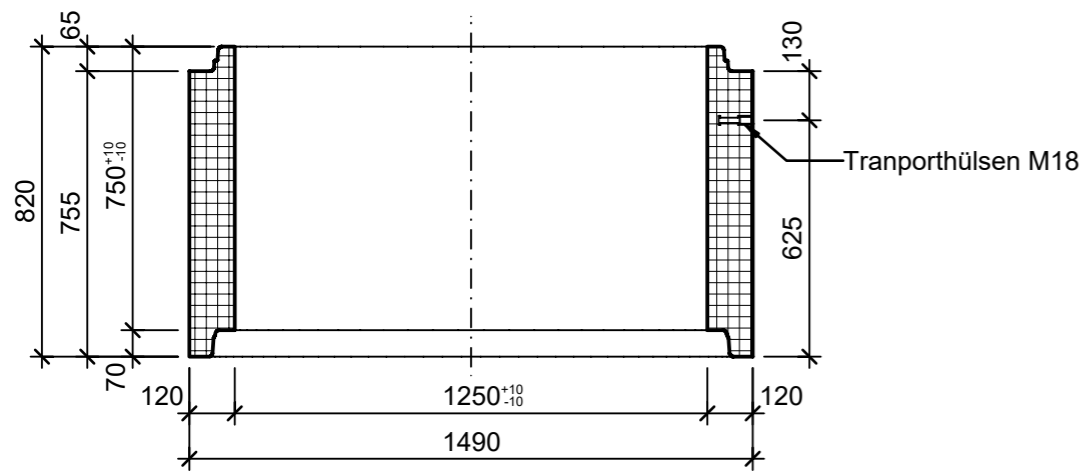
Schnitt 1-1, 1:20
