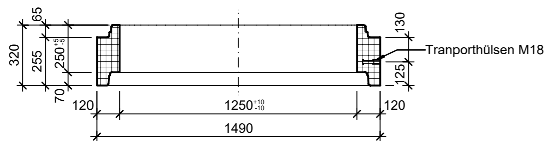
Schnitt 1-1, 1:20
