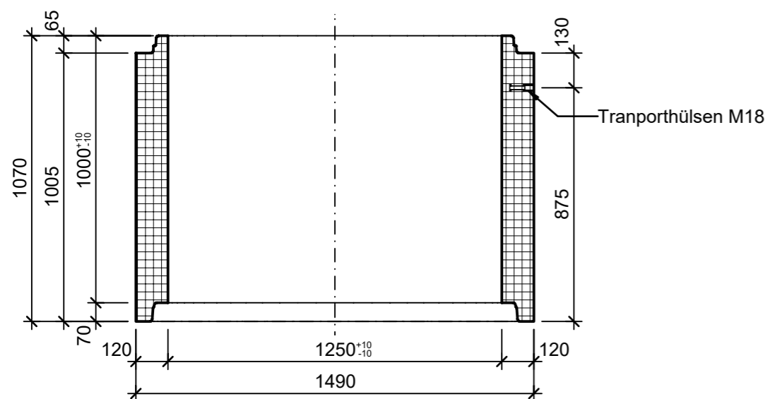
Schnitt 1-1, 1:20
