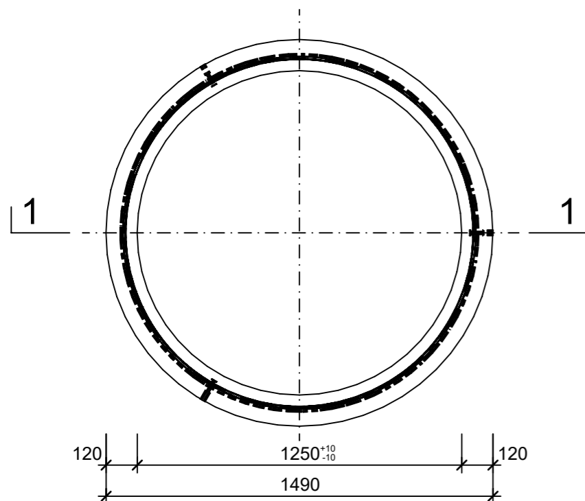
Grundriss, 1:20
