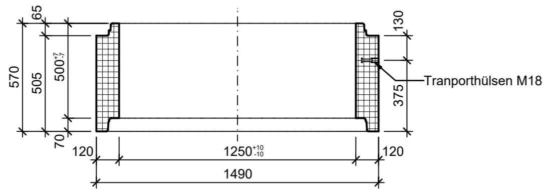
Schnitt 1-1, 1:20
