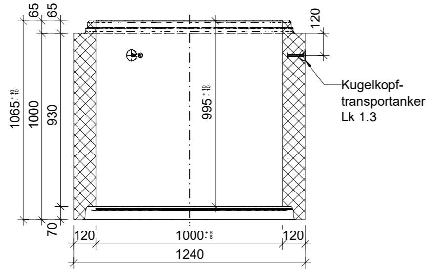
Schnitt 1-1, 1:20
