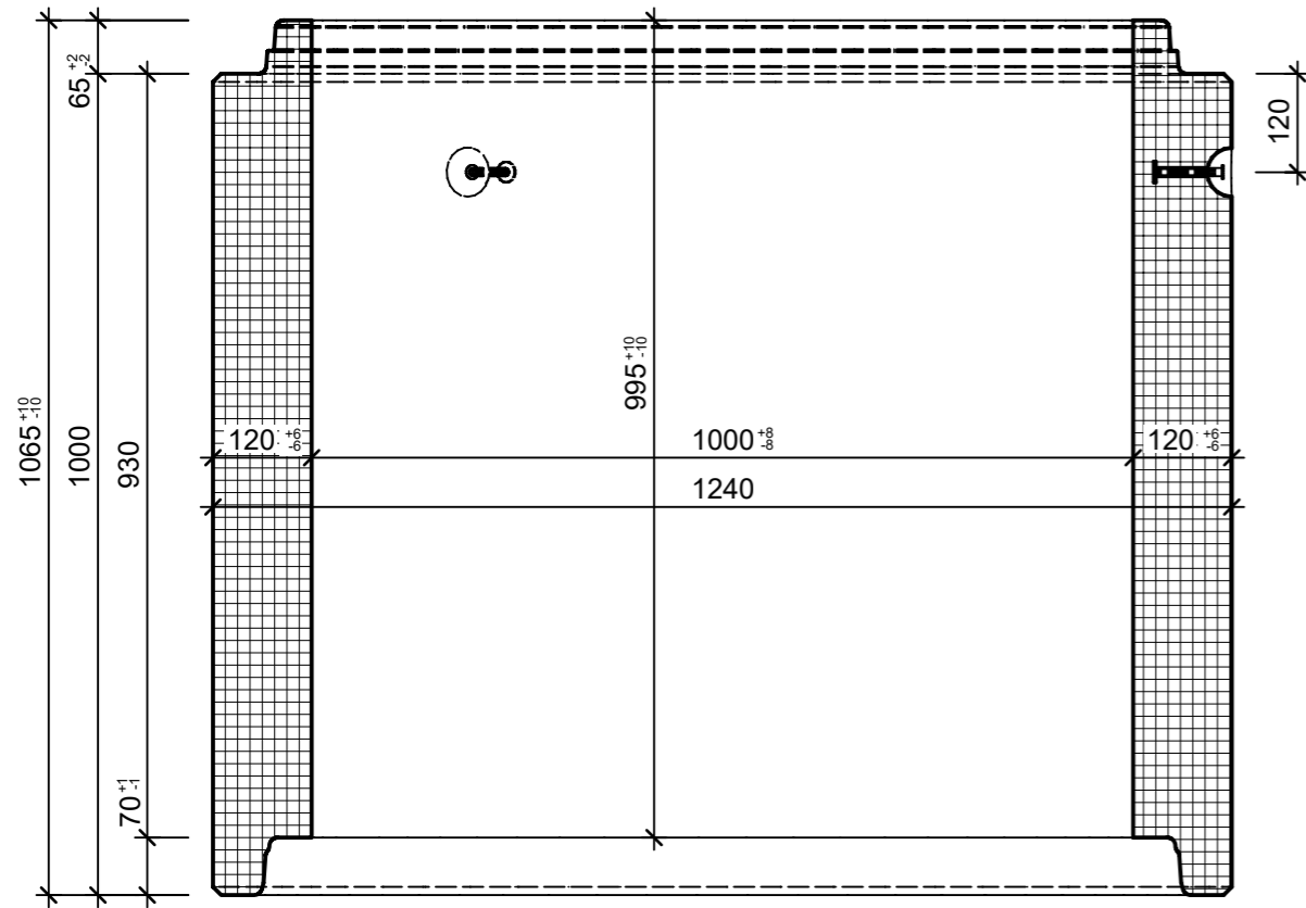
Grundriss, 1:10
