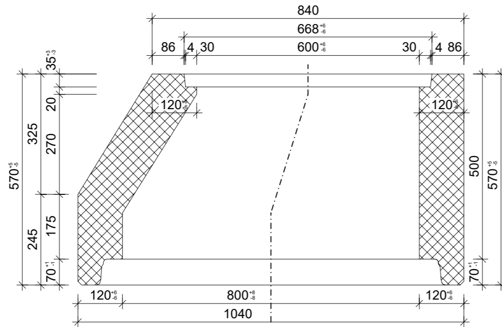
Schnitt 1-1, 1:10
