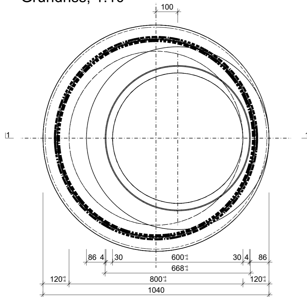
Grundriss, 1:10
