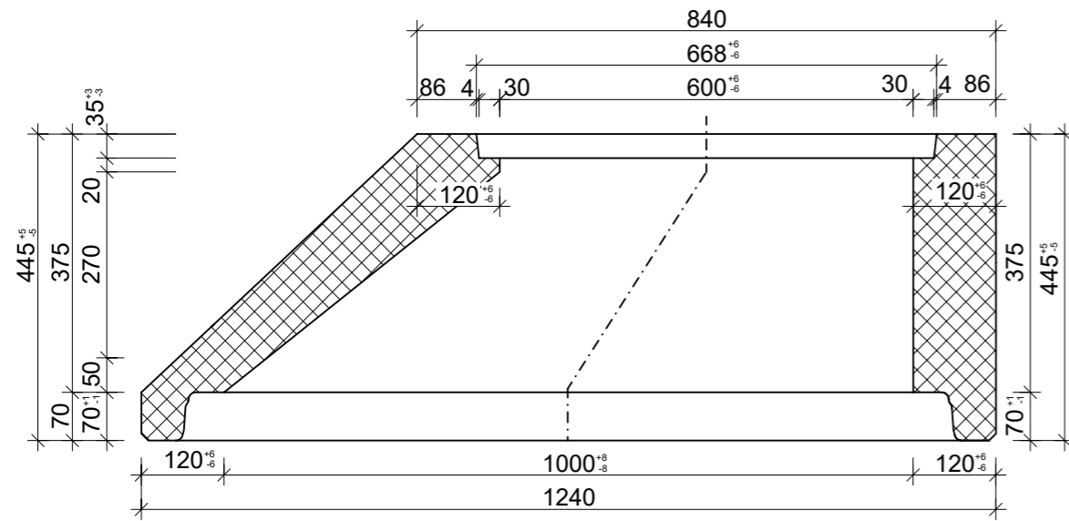
Schnitt 1-1, 1:10
