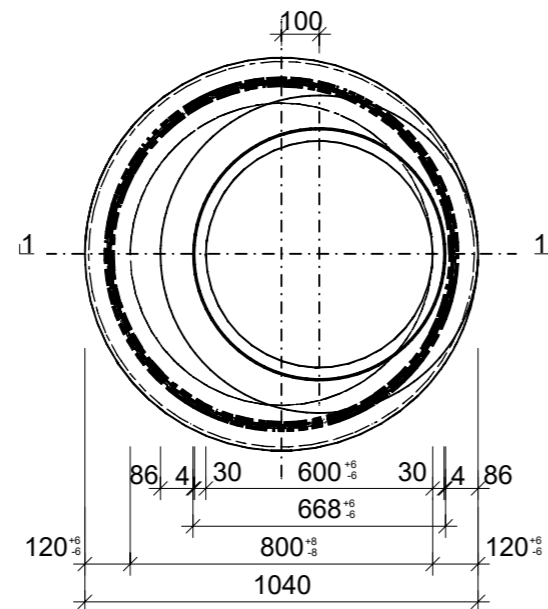
Grundriss, 1:20
