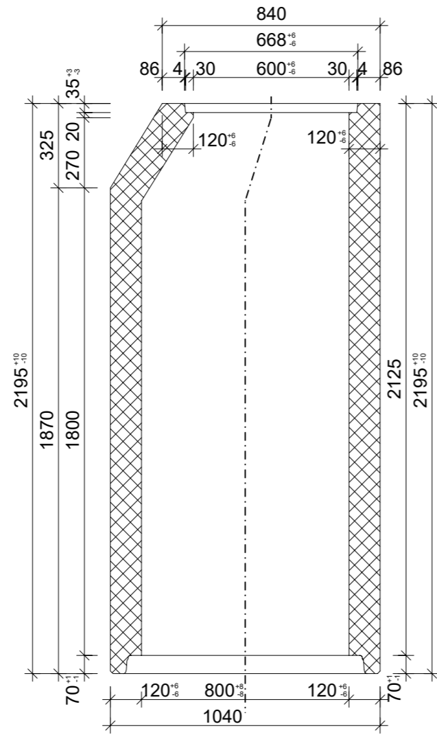
Schnitt 1-1, 1:20
