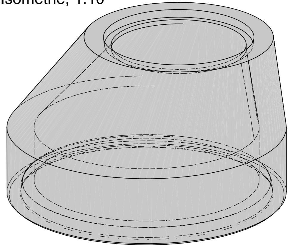
Isometrie, 1:10
