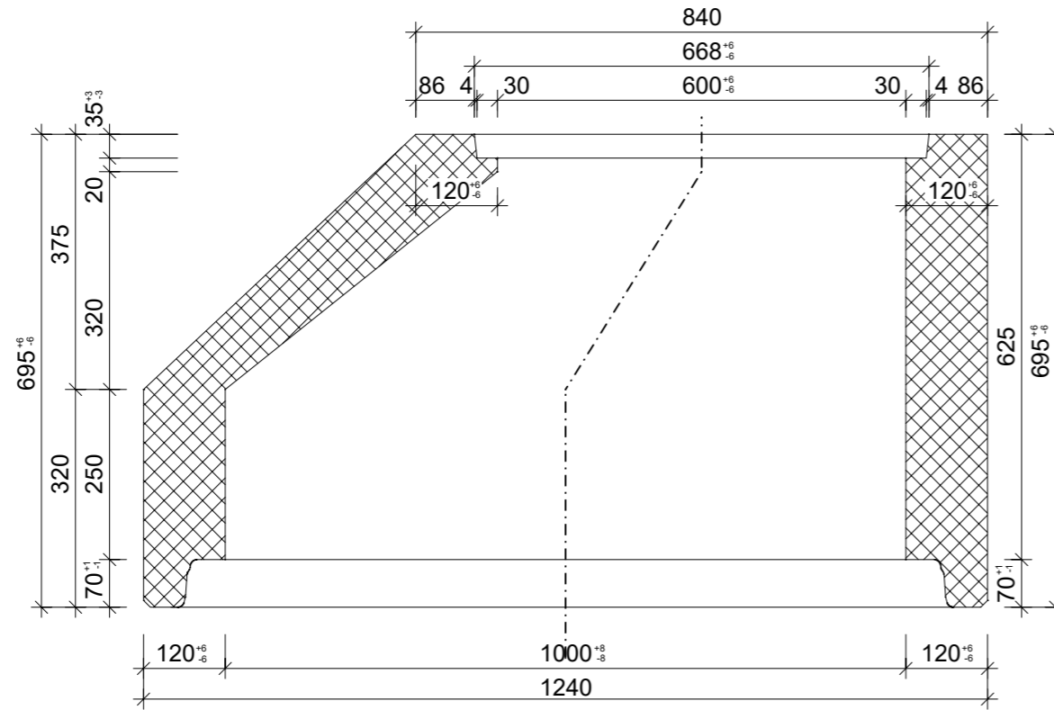
Schnitt 1-1, 1:10
