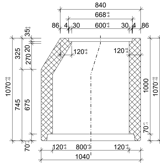
Schnitt 1-1, 1:20
