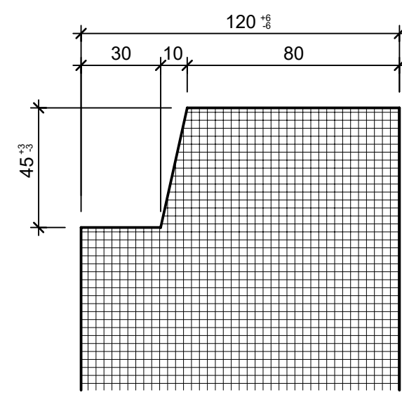
Detail A, 1:2
