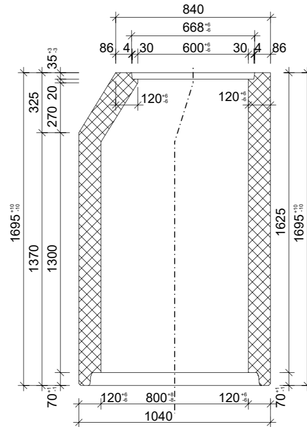
Schnitt 1-1, 1:20
