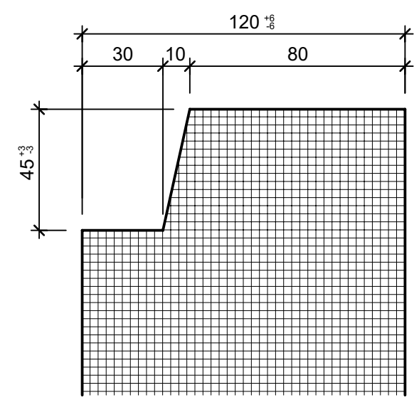
Detail A, 1:2
