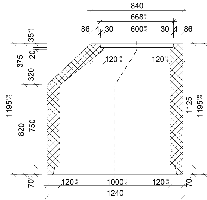
Schnitt 1-1, 1:20
