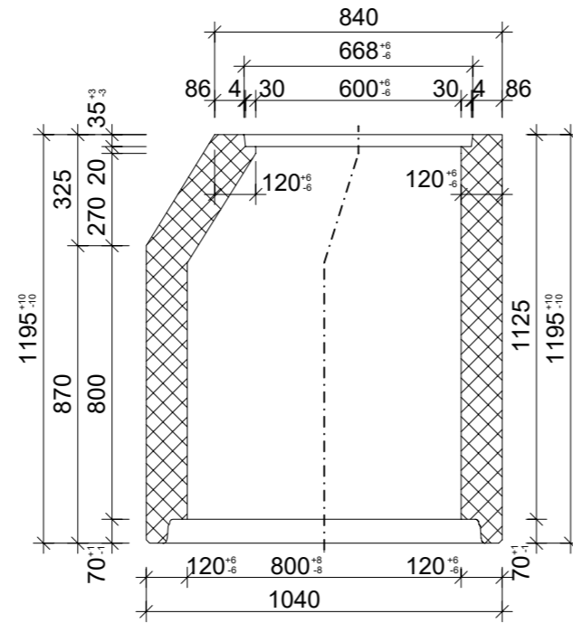
Schnitt 1-1, 1:20
