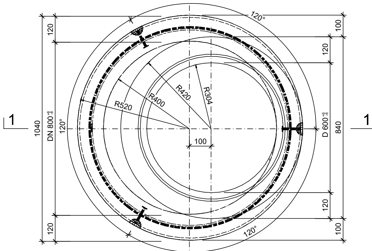
Grundriss, 1:10
