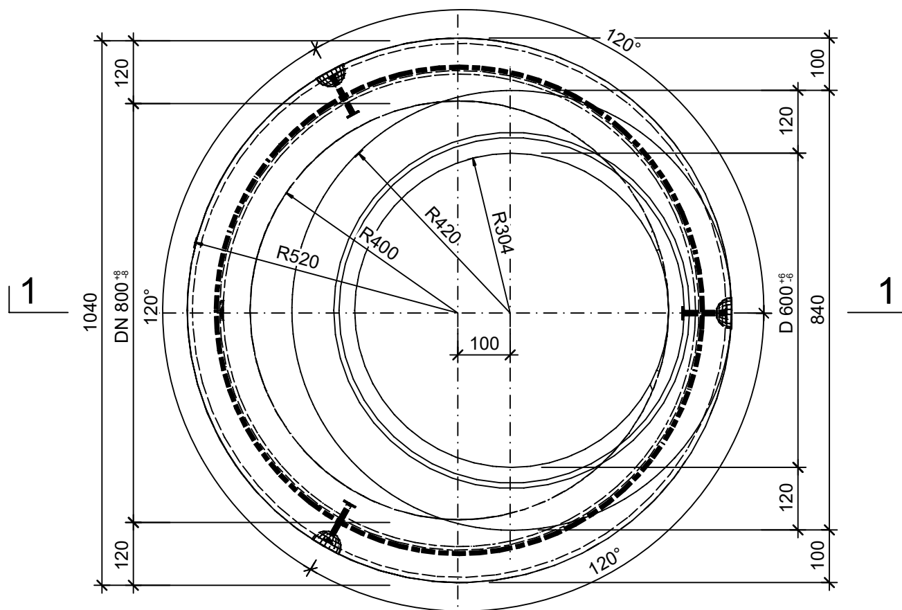
Grundriss, 1:10
