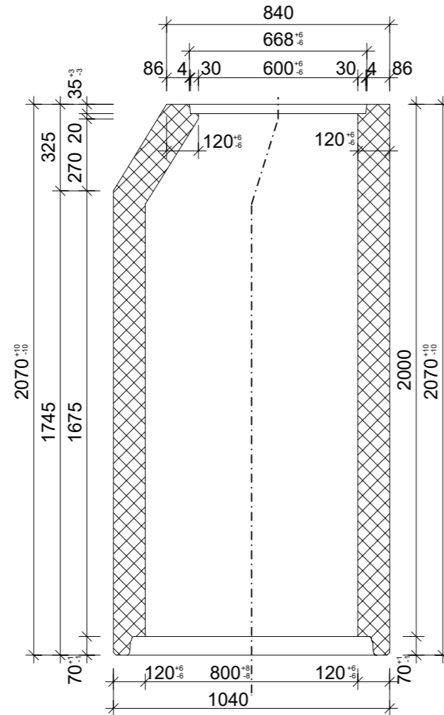
Schnitt 1-1, 1:20
