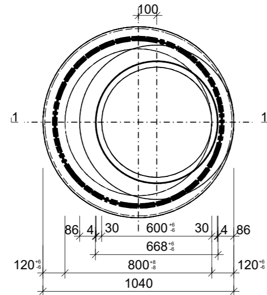
Grundriss, 1:20
