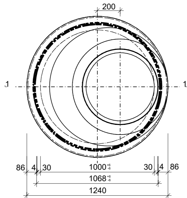
Grundriss, 1:20
