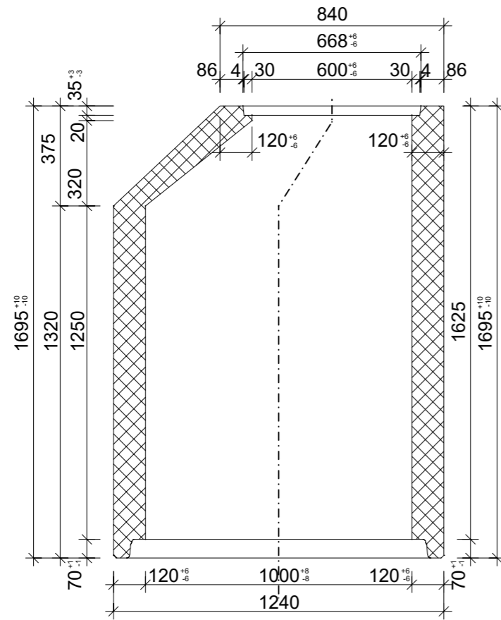
Schnitt 1-1, 1:20
