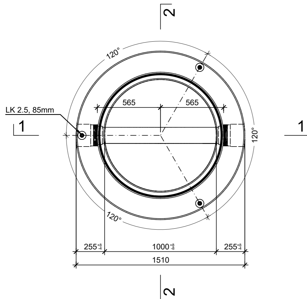
Grundriss, 1:20
