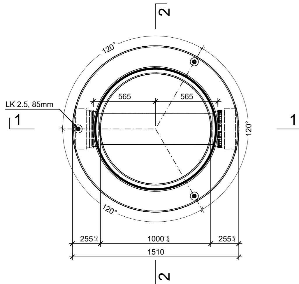
Grundriss, 1:20
