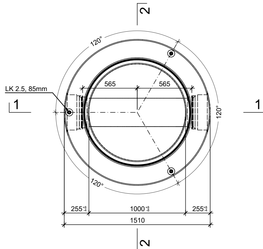
Grundriss, 1:20
