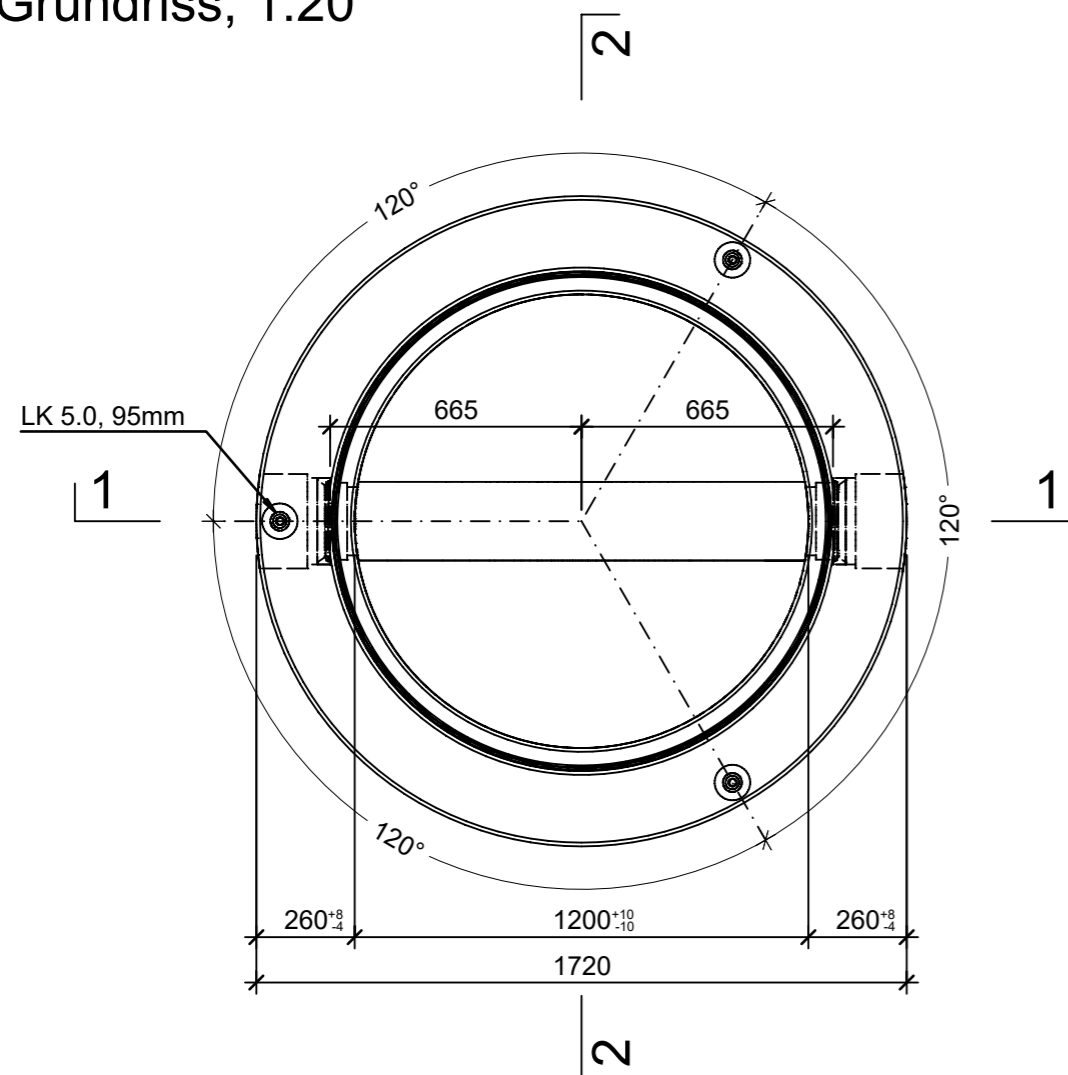
Grundriss, 1:20
