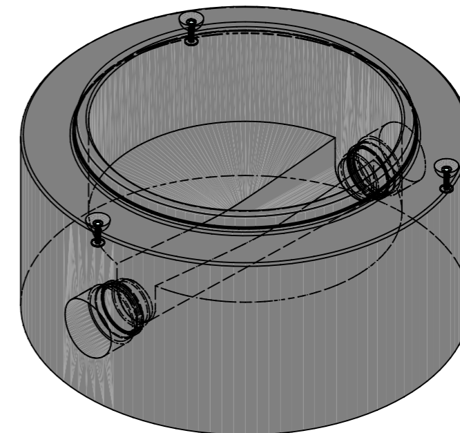
Isometrie
