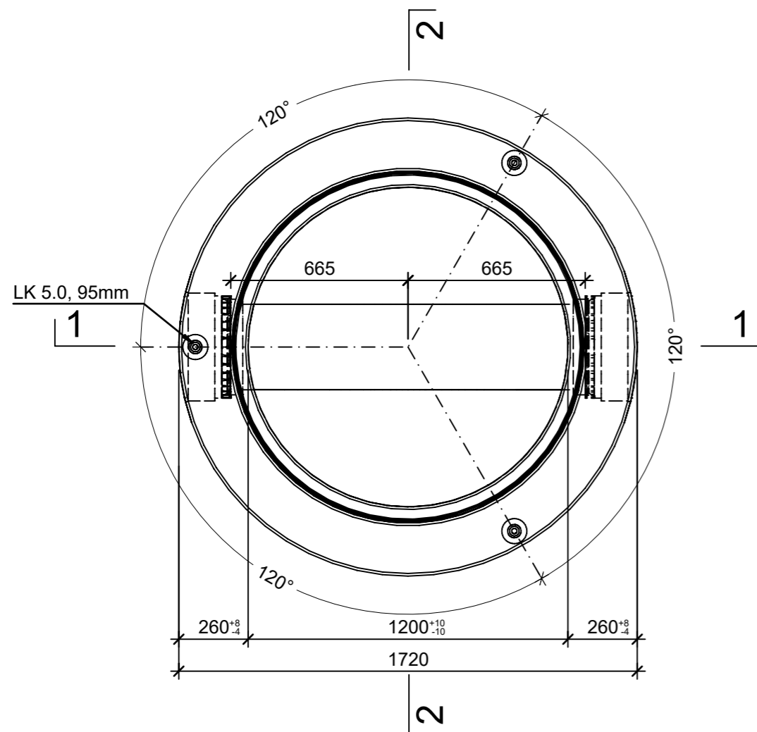
Grundriss, 1:20
