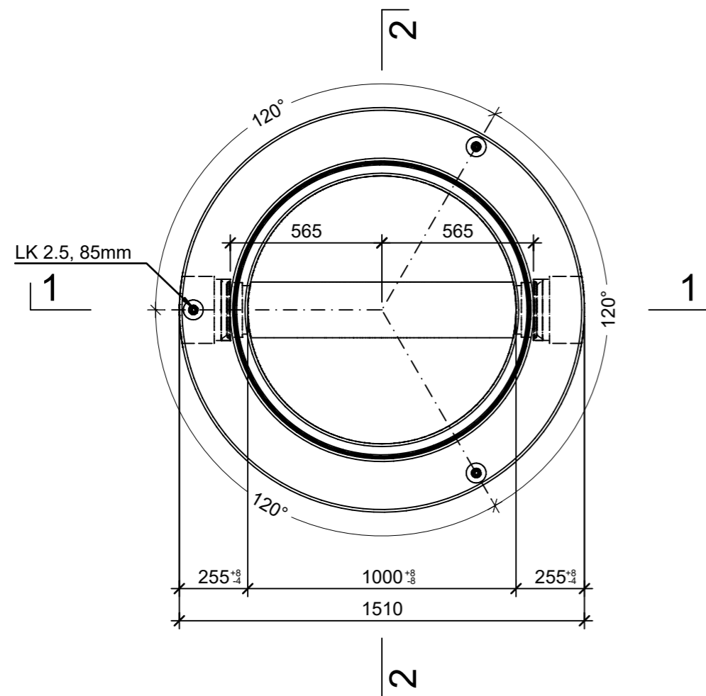
Grundriss, 1:20
