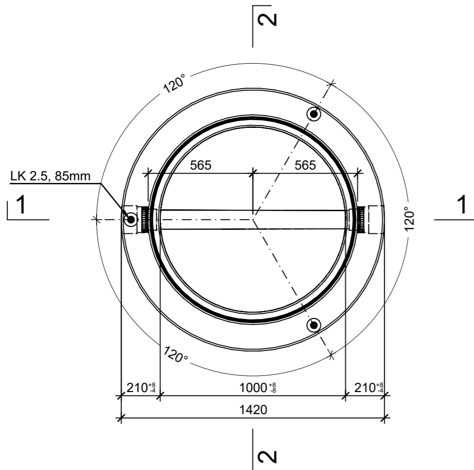
Grundriss, 1:20
