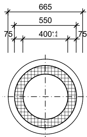
Schnitt 1-1, 1:20
