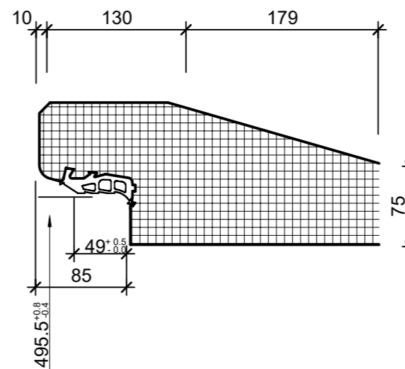
Detail Glockenmuffe, 1:5
