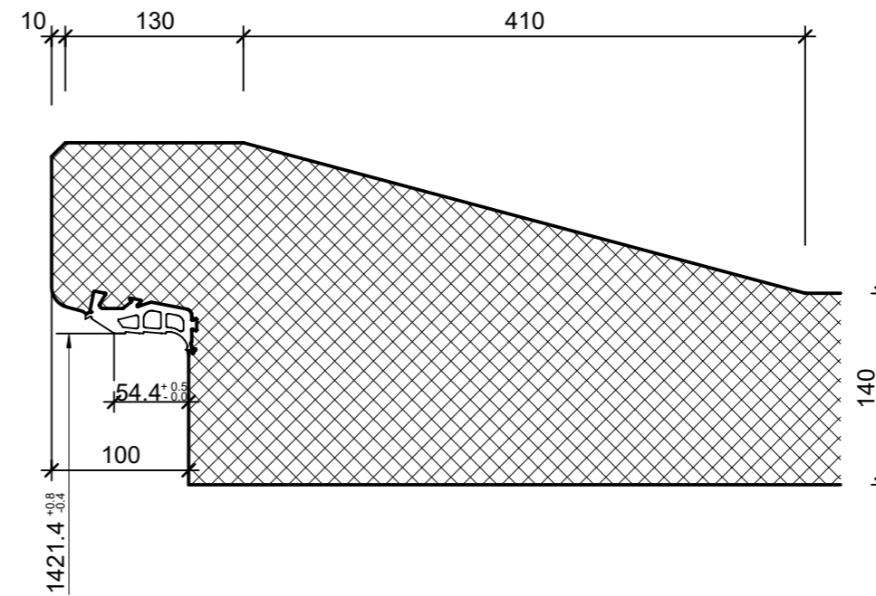
Detail Glockenmuffe, 1:5
